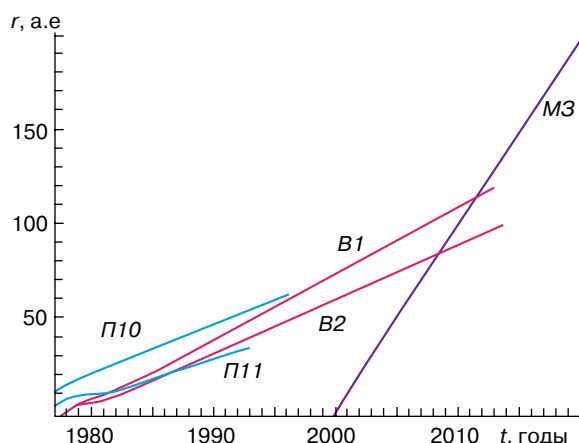
Рис. 1. Гелиоцентрическое расстояние r американских космических аппаратов “Вояджер-1” ( B1 ), “Вояджер-2” ( B2 ), “Пионер-10” ( П10 ) и “Пионер-11” ( П11 ) как функции времени. Показана также траектория космического аппарата “Межзвездный зонд” ( M3 ) (предполагаемый запуск в США в 1999 году).
